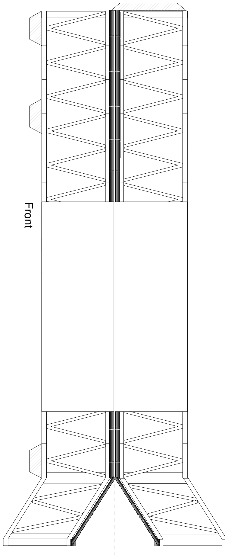
Blatt 15 Geländer Plattform: Front und 45 Grad-Ecke hinten
